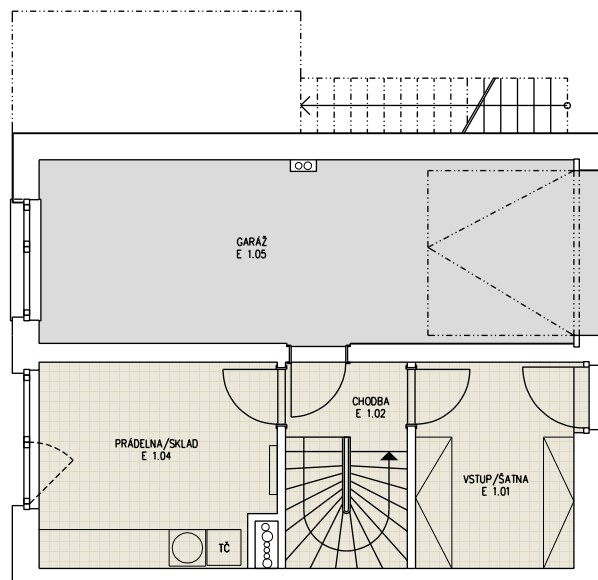
Podlaží: 1.NP
